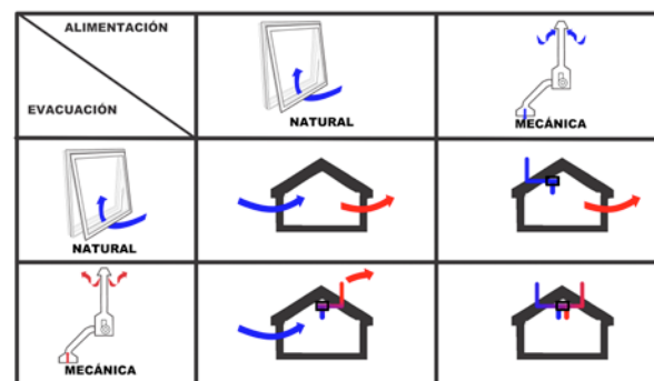
Figura 9.17: Tipos de alimentación y evacuación de aire
