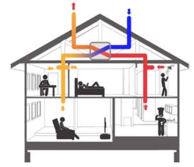
Figura 9.12: Esquema de ventilación con recuperador de calor
