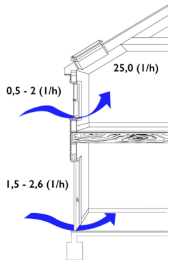
Figura 6.3: Infiltración de aire en ventanas y puertas en viviendas de madera.
