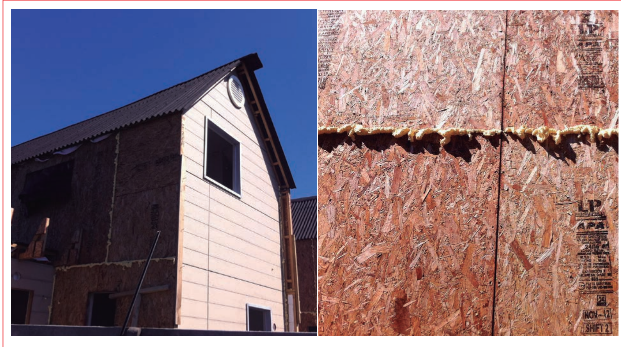
Figura 10.11: Sellos de poliuretano inyectado en uniones entre placas de OSB
