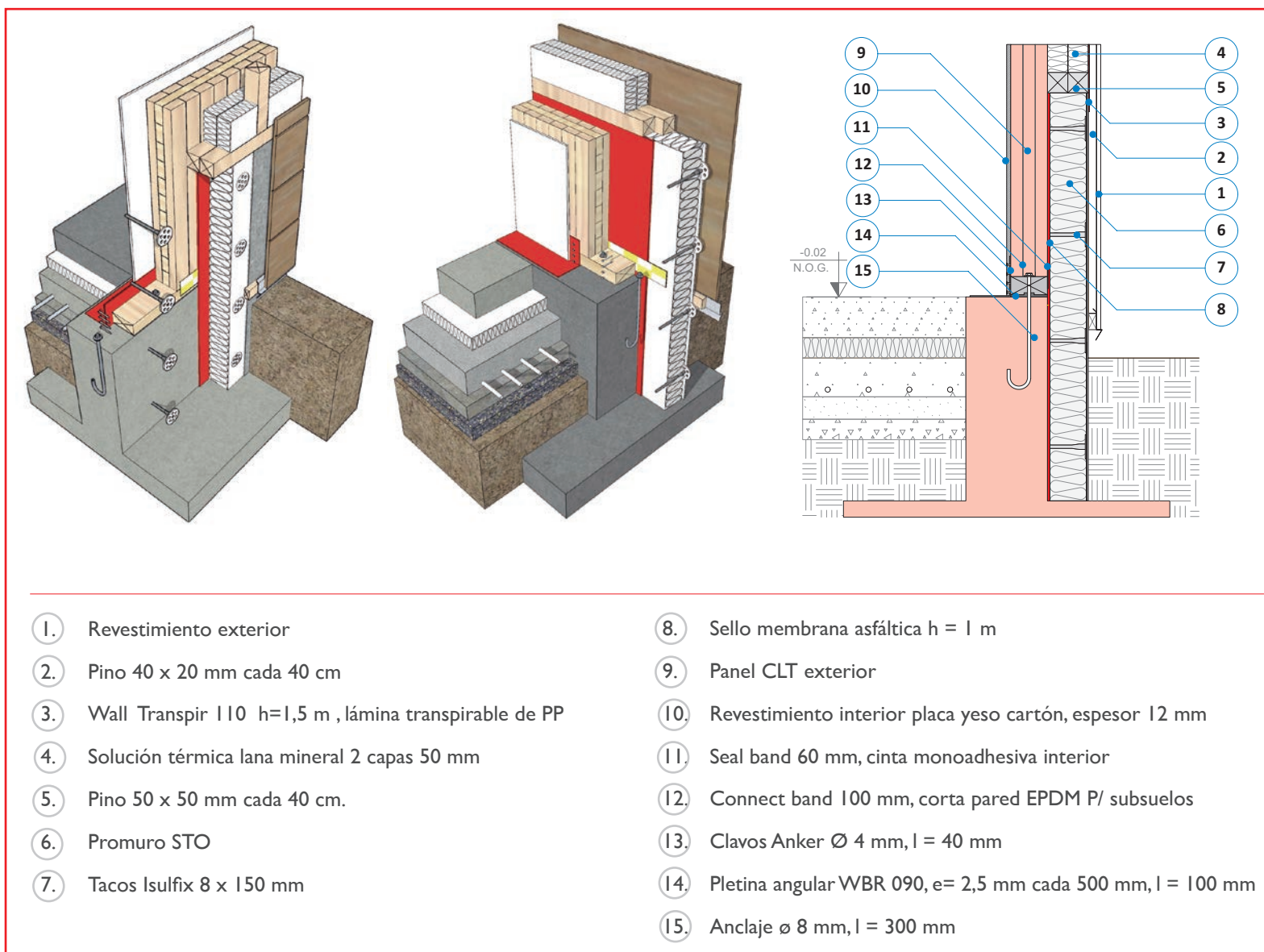
Figura 10.28: Detalle unión entre el muro y el sobrecimiento
