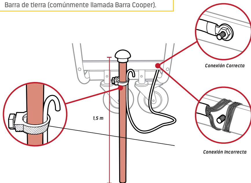
f.05_ Barra de tierra (comúnmente llamada Barra Cooper).
