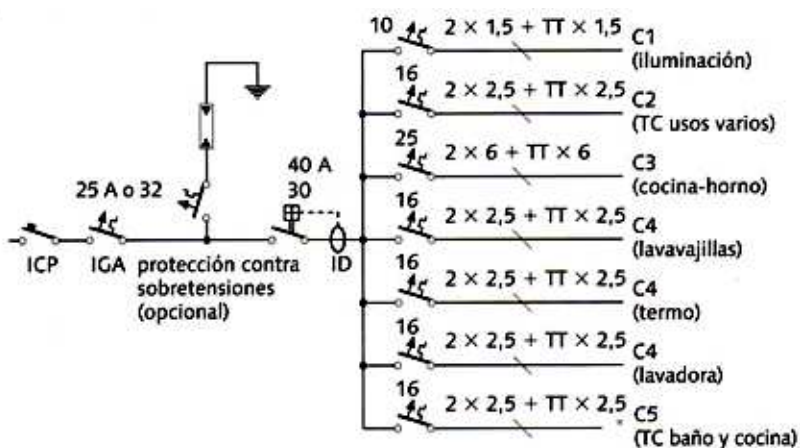
Simbología interruptores del CGMP
