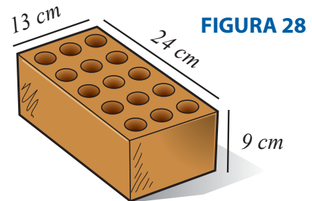
LADRILLO “KING KONG 18 HUECOS”, USADO PARA LOS MUROS PORTANTES.
